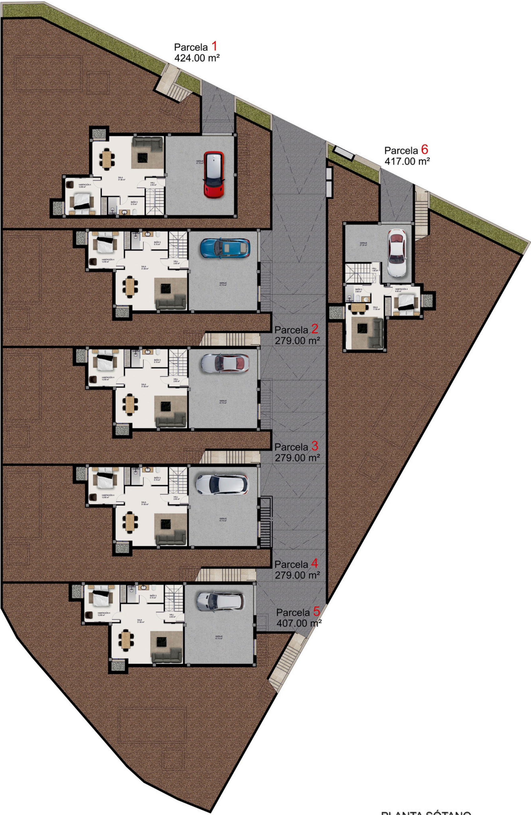
PLANTA SÓTANO
